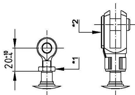
Abbildung 6: Kolbenstangenaufhängung
